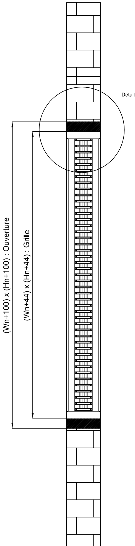
GE60 XL - grilles de ventilation 3 et 4
